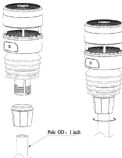
Abbildung 4: Montage Außensensor
